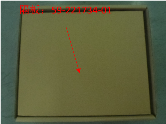
再盖上最后一块隔板(这是第三块隔板)
